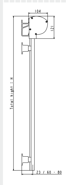
Vidar Screen i profil
