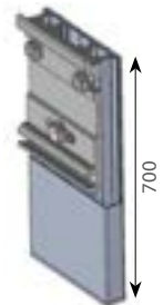
Lodrät monteringsplatta för vägg inkl. standardbeslag. Se sid 36 för ytterligare info om mått och montering.
