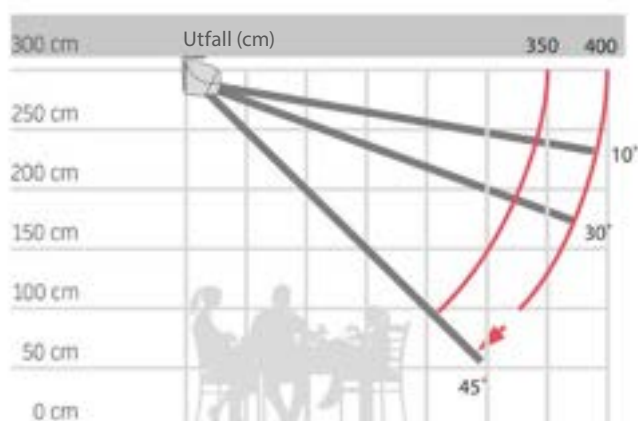
Montering tak
