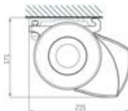
Takmontering
