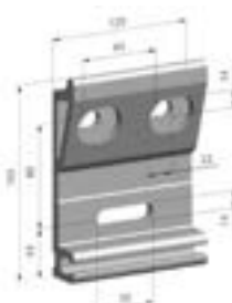
Specialbeslag tak/vägg
