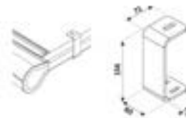
U-monteringsvinkel takmontage 156x71 mm
