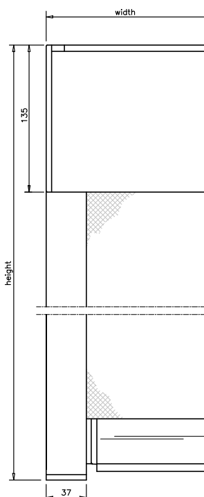
Beaufort® Zip 135
