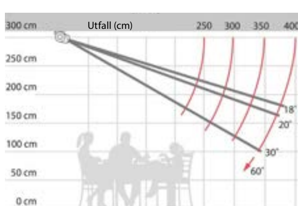
Montering tak
