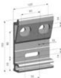
Specialbeslag tak/vägg
