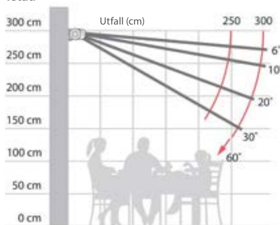
Montering vägg
