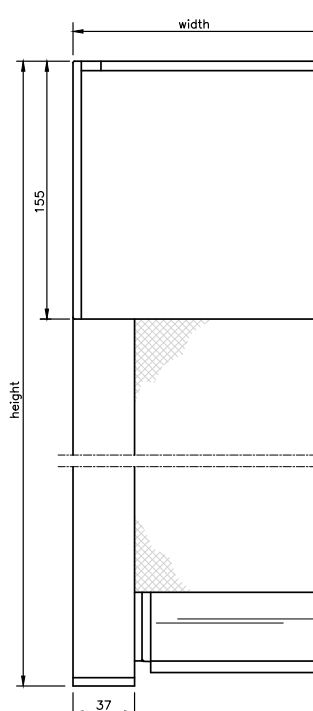
Beaufort® Zip 155
