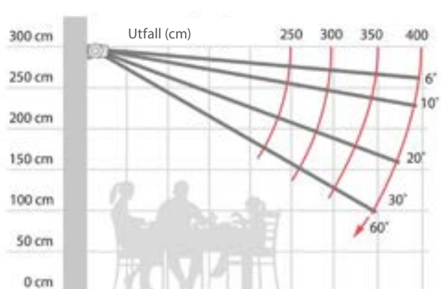
Montering vägg
