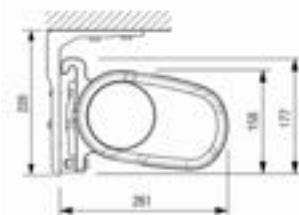
Takhöjning med L-vinkel
