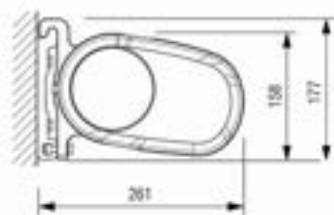
Vägghöjning
