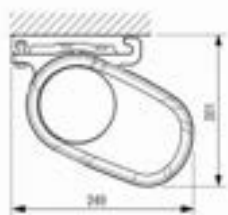
Takhöjning
