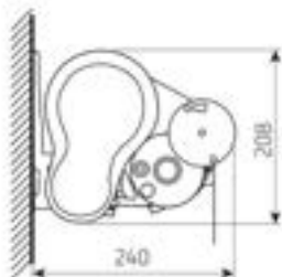
Bergen Öppen Vägghäring
